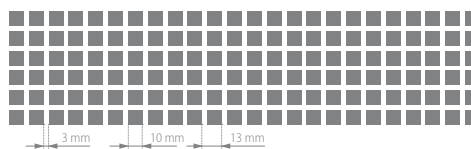
CG - 5 BESCHICHTUNG - 59%
